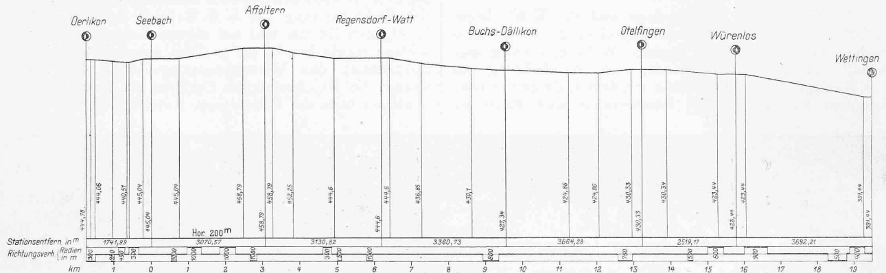
Abb. 2. Längenprofil der Linie Seebach-Wettingen.
