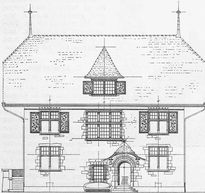
Fig. 11 et 12. Deux façades de la villa Jäger à Lausanne. — Echelle 1 : 200. — Architectes MM. Schmid et Rosset, Lausanne et Veveytaux.
