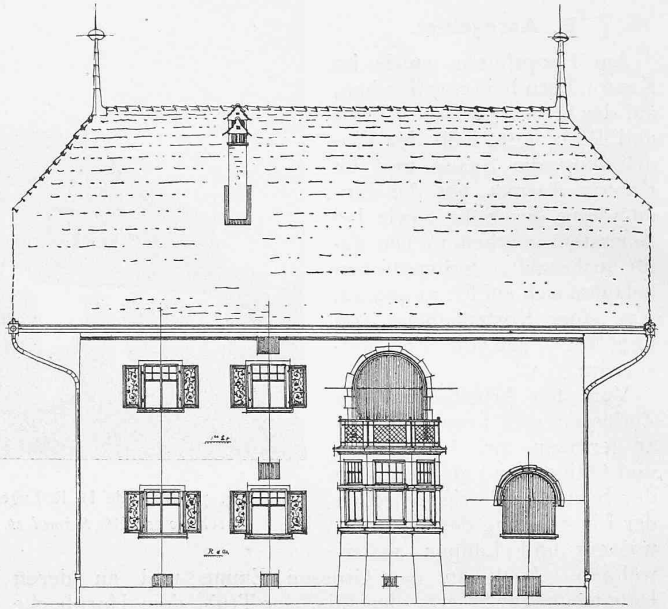
Fig. 11 et 12. Deux façades de la villa Jäger à Lausanne. — Echelle 1 : 200. — Architectes MM. Schmid et Rosset, Lausanne et Veveytaux.
