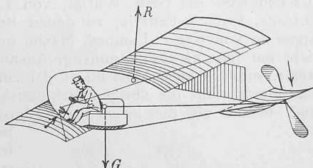
Abb. 20. Automatisch stabiler Drachenflieger (mit Weglassung der Anlaufräder).
