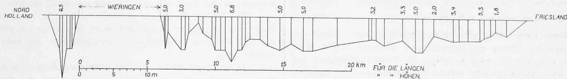
Abb. 3. Längsprofil des Abschlussdammes. — Masstab 1 : 250 000 für die Längen, 1 : 500 für die Höhen.
