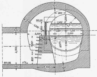
Abb. 16. Ueberlauf bei Fenster Nr. 2 zur Regulierung des Wasserzulaufes.
