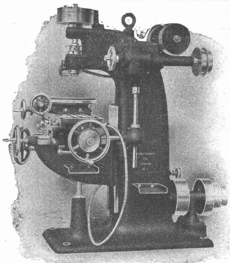
Vertikal-Fräsmaschine „Herbert“ No. 1.
