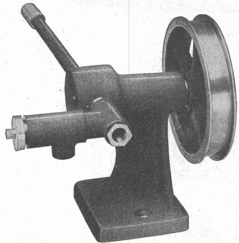
Flügelpumpe für Oel und Seifenwasser.
