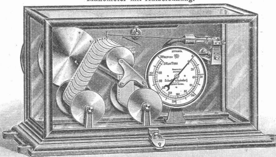
Manometer mit Aufzeichnung.
