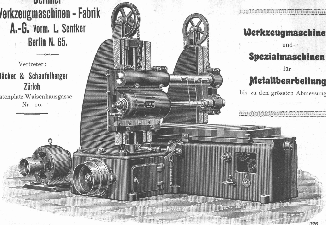
Langfräsmaschine.
