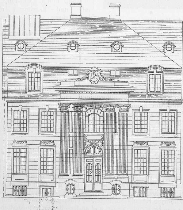
Abb. 26. Familienhaus an der Hartstrasse. — Strassenfassade. Masstab 1 : 200.
