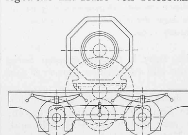
Abb. 19. Anordnung von Gestellmotoren mit Zahnradübersetzung der Thomson-Houston Co. von 1890 und der Maschinenfabrik Kraus & Cie. von 1895. Masstab 1 : 50.
