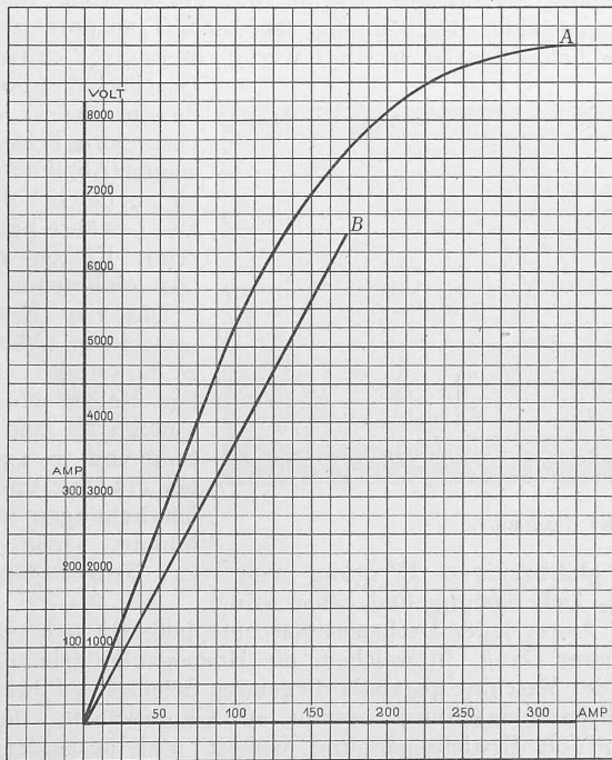
Abb. 33. Garantiekurven des Generators. Legende: A Leerlaufkurve, B Kurzschlusskurve.
