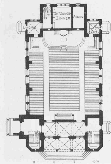
Abb. 1. Grundriss der Kirche. Maßstab 1 : 500.
