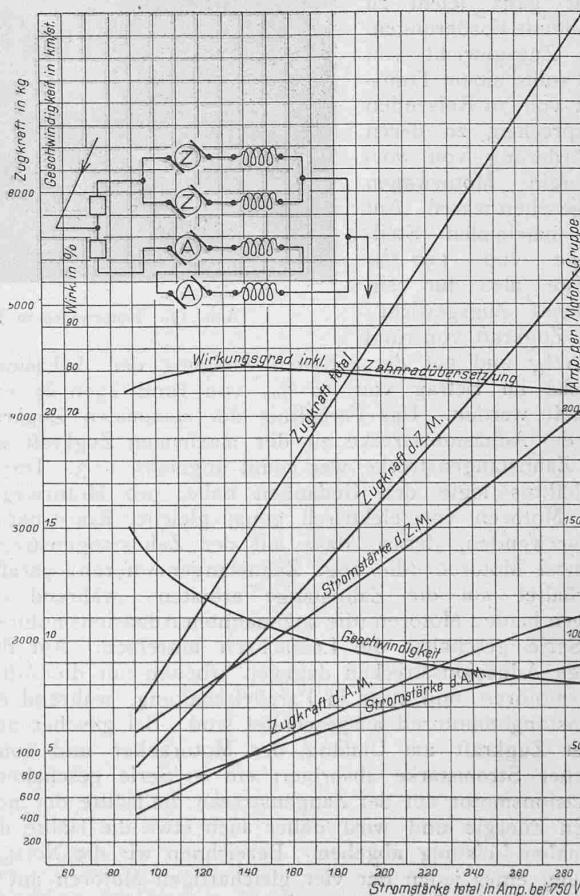
Abb. 20. Motorkurven und Schema der Motorenschaltung auf der Zahnstangentrecke.
