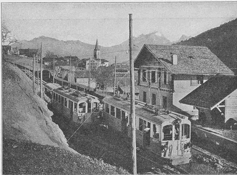
Abb. 26. Zugskreuzung auf der Station Troistorrents.
