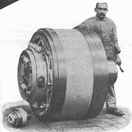
Benn Kupplung Nr. 12 für 650 P.S. geliefert in eine Zementfabrik.
