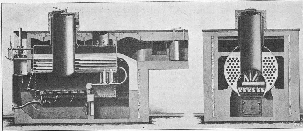
Abb. 29. Schmeldeiserner Kessel für Niederdruckdampf-Heizung von Gebr. Sulzer, Winterthur. — Masstab 1:50.
