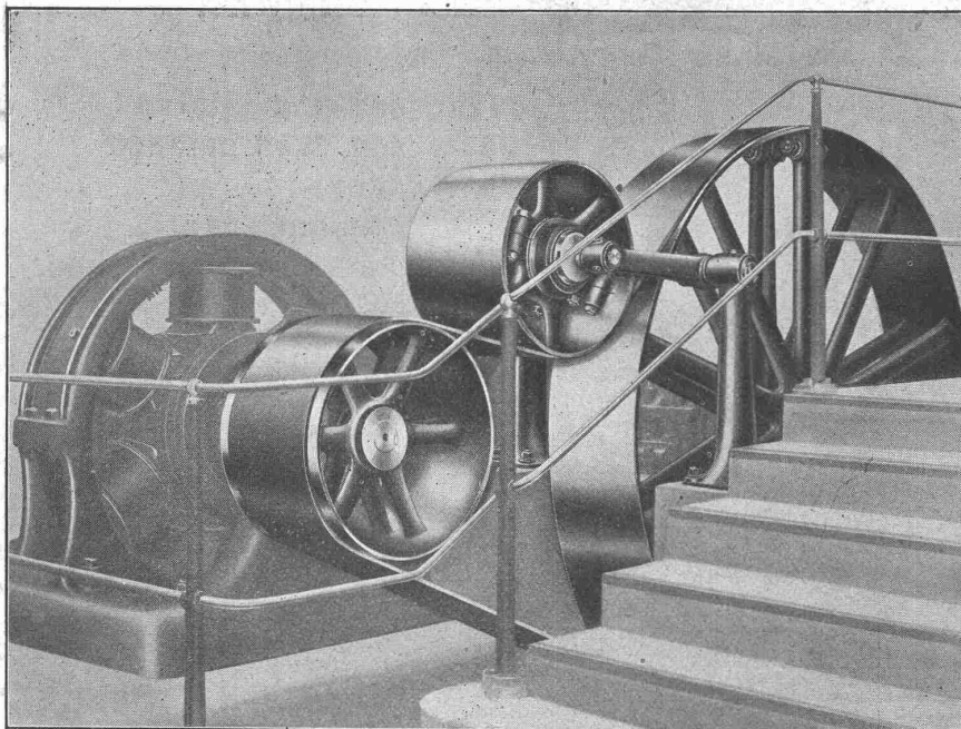
Spannrollentrieb mit Oelumlauf geliefert für Generator-Antrieb 225 P. S. 500 mm breiter Doppelriemen.
