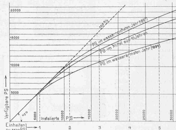
Abb. 2. Charakteristische Kurven.
