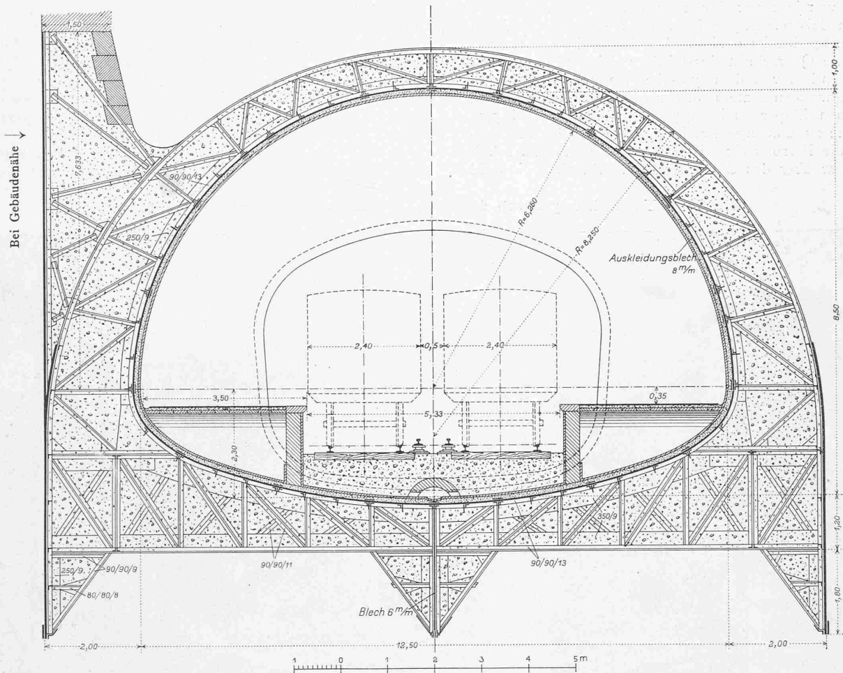
Abb. 10. Querschnitt durch einen der 16,5 m breiten und 66 m langen Caissons für die Stationsstrecken. — 1 : 100.
