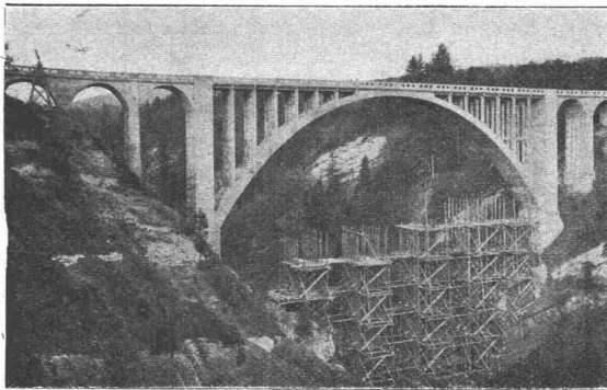
Gmündertobelbrücke; grösster Bogen in armiertem Beton von 79 m Spannweite. Völlendet 1908.
