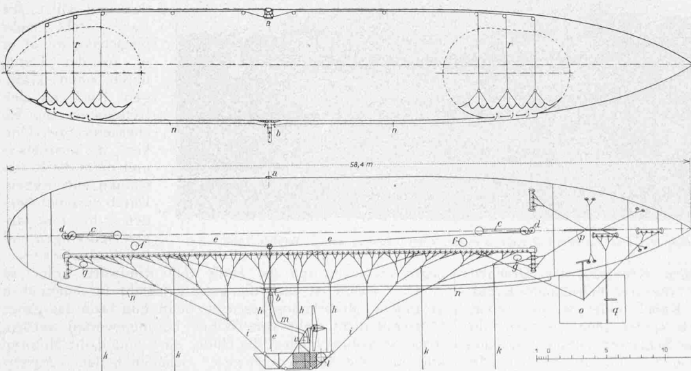
Abb. 4 und 5. Seiten- und Vorderansicht, sowie Längsschnitt durch die Hülle des Parseval-Luftschiffes «Modell E».
