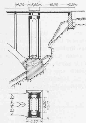
Variante für die Widerlager. Masstab 1 : 750.
