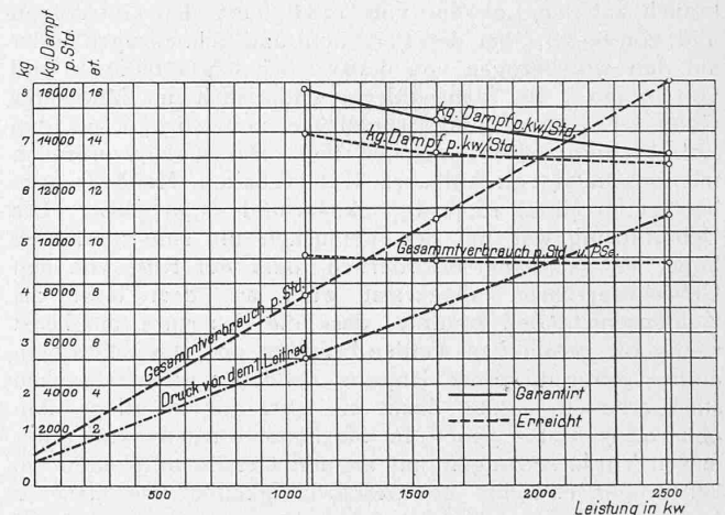
Schaulinien der Versuchsgruppe IV (2300 kw).
