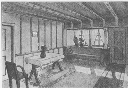
Grundrisse vom Keller, Erdgeschoss und I. Stock. Schnitt und Westfassade. Innenansicht der Diele in der Wohnung des Arztes. Masstab 1:800.
