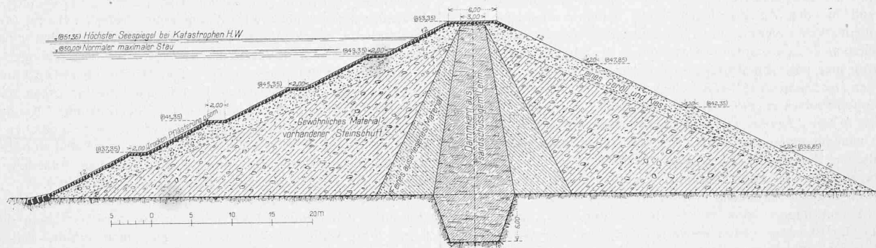
Abb. 11. Normalprofil des Staudammes am Klöntalersee. — Masstab 1:600.
