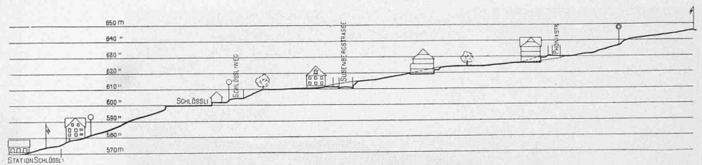
Querschnittsprofil des Schlössli-Susenbergs-Areals (Profil V zum Entwurf Pflughard & Häfeli). — Masstab 1:3000.
