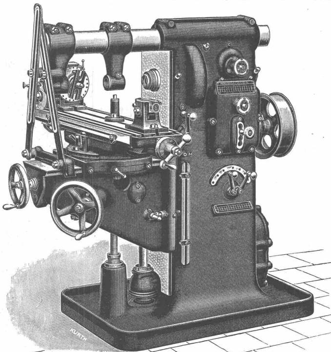
Wanderer-Rapid-Fräsmaschine Nr. 2 mit Einzelscheiben-Antrieb.
