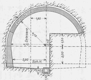
Abb. 6. Profile der Rampentunnel mit und ohne Verkleidung. — 1:200.
