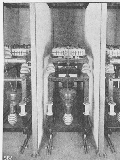
Abb. 102. Ausschaltbare Wurz-Blitzschutzapparate, 27000 Volt.
