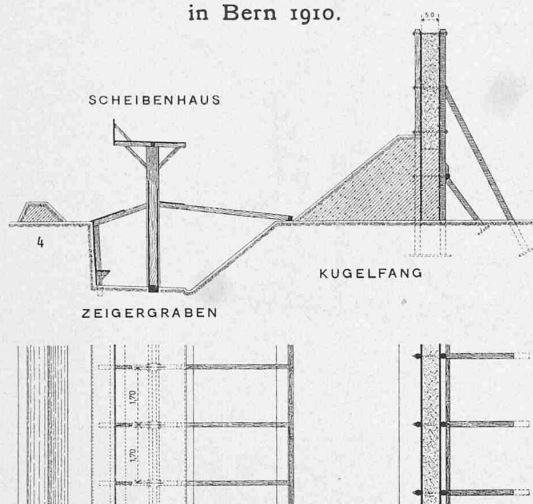
Abb. 10. Schnitte und Grundriss vom Scheibnhaus und Kugelfang. Masstab 1 : 200.
