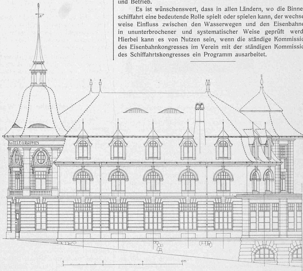
Abb. 6. Fassade gegen die Avenue William Frasse. — Masstab 1:250.
