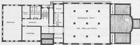
Grundrisse vom Untergeschoss, Erdgeschoss und Obergeschoss. — 1:800.
