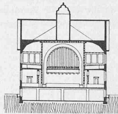
Querschnitt 1:800.
