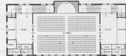
Grundrisse vom Obergeschoss und Dachgeschoss. — 1:800.
