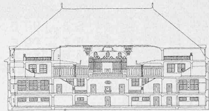
Längsschnitt. — Masstab 1:800.
