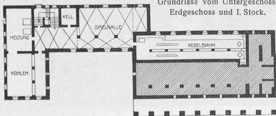
Masstab 1 : 800.
