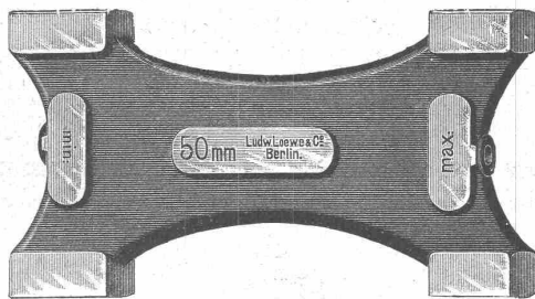
Toleranz-Flachkaliber Mba.
