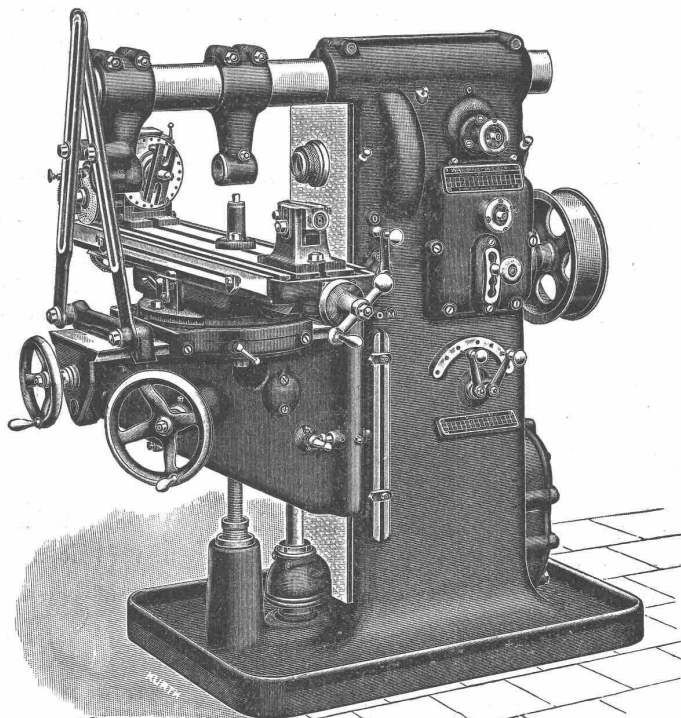
Wanderer-Rapid-Fräsmaschine Nr. 2 mit Einzelscheiben-Antrieb.
