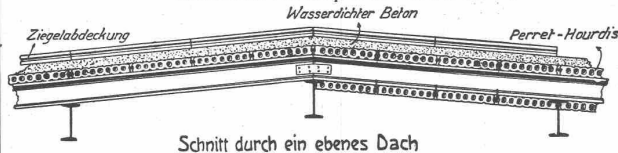
Schnitt durch ein ebenes Dach
