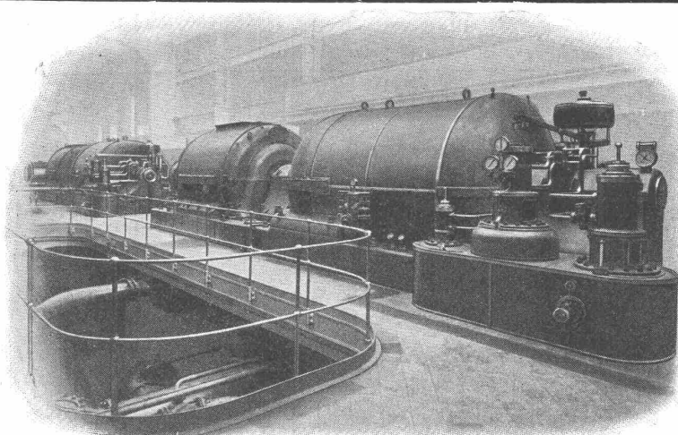
10000 PS Oerlikon-Turbogeneratoren im Elektrizitätswerk Stockholm
