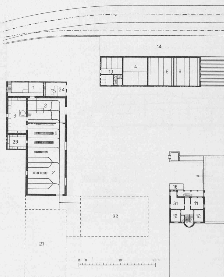
Grundrisse, Schnitte und Ansichten. — Masstab 1:600.
