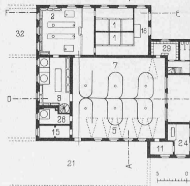
Grundriss und Schnitte. — Masstab 1:600.
