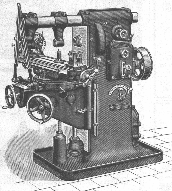
Wanderer-Rapid-Fräsmaschine Nr. 2 mit Einzelscheiben-Antrieb.
