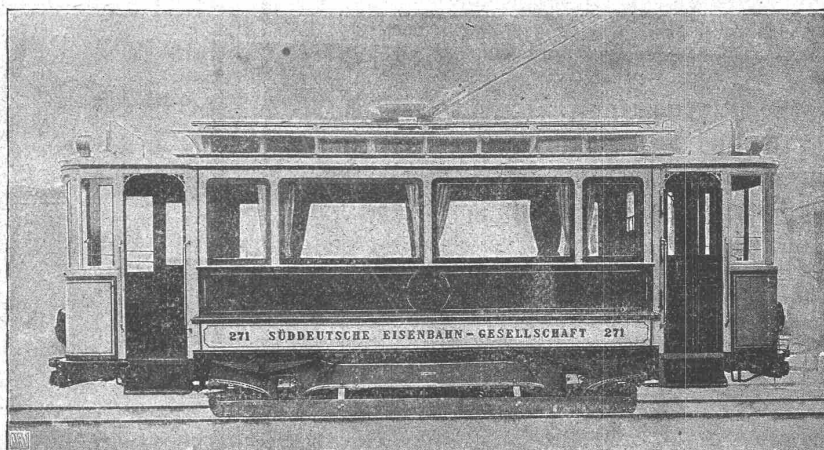
Motorwagen mit 20 Sitz- und 15 Stehplätzen. Type: Mit Längssitzen, mittlere Seitenfenster herablassbar. Plattformen mit vorderer Verglasung und seitlich mit Flügeltüren, vollständig abschliessbar; Radstand 3,2 m.
