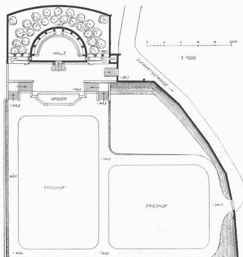
Lageplan von Friedhof und Halle
