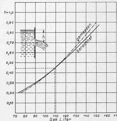
Abbildung 8. Wassermengenkurven.
