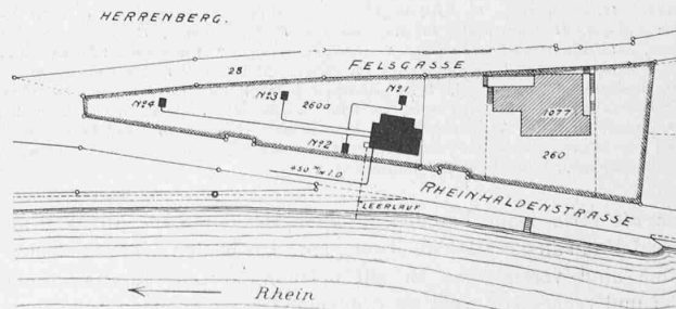
Abb. 2. Lageplan des Pumpwerks Rheinhalde. — 1:2000.
