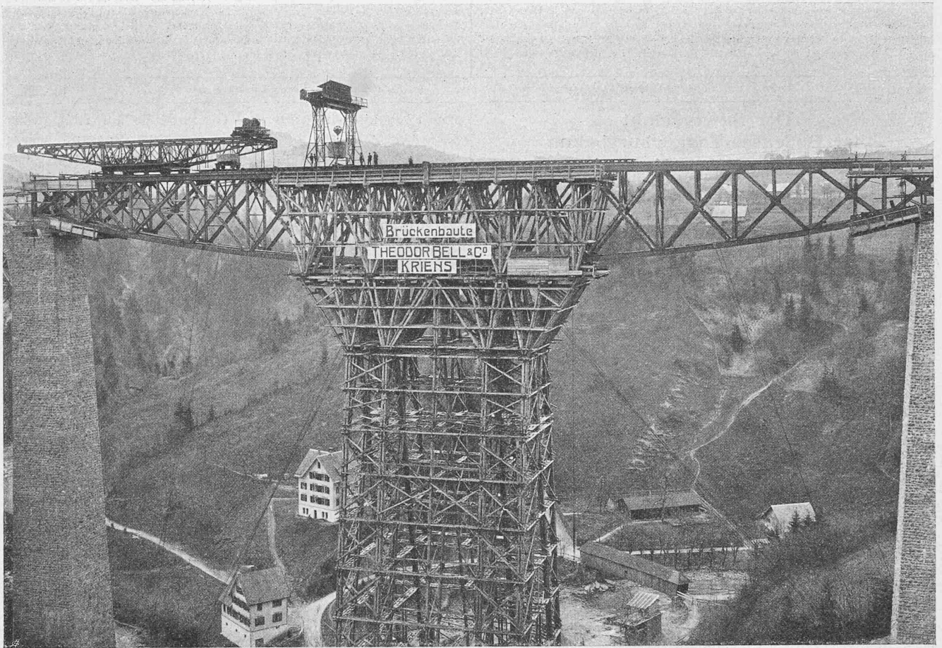
Abb. 56. Oberer Teil des Gerüstturms, Montage nahezu vollendet, Aufziehen der 7. Auflagerquader mittels des Hubkrans im April 1910.
