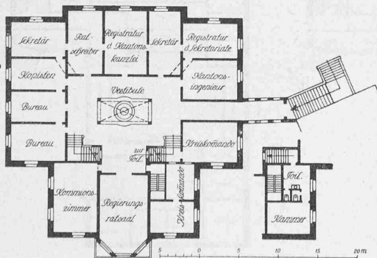
Grundrisse vom Keller, Erdgeschoss, I. Stock und Obergeschoss. — Masstab 1:600.
