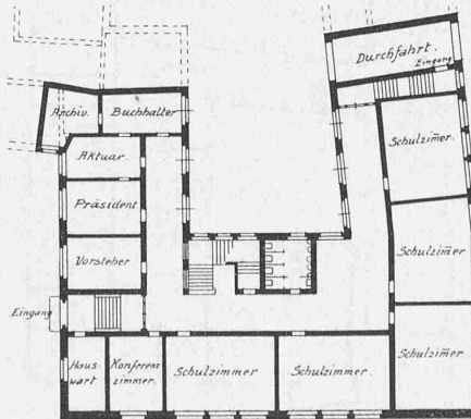
Südfassade und Haupteingang. Grundrisse vom Erdgeschoss, I. Stock und Dachstock. — 1:600.
