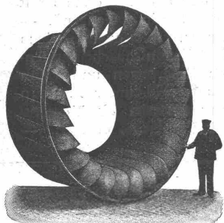
Laufgrad einer Francis turbine von 740 HP, 3,8 m Diameter, 10 000 kg
