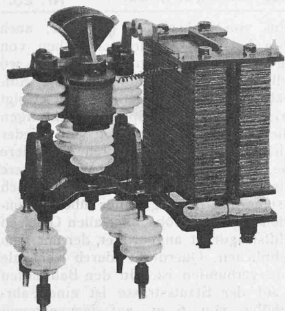
Abb. 11. Hörnerblitzschutz-Apparat.
