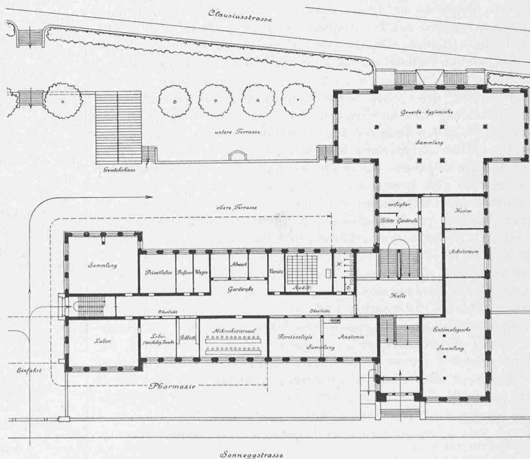
Sammlungsgebäude an der Sonneggstrasse. — Grundriss des obern Erdgeschosses. — 1 : 800.
