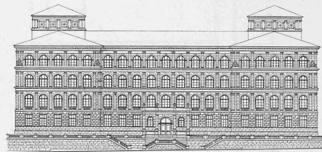
Entwurf Nr. 5. „Dominante.“ — Querschnitt durch das Sammlungsgebäude an der Sonneneggstrasse. — 1:800. — Fassade gegen die Clausiusstrasse.
