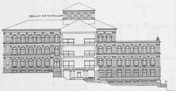
Entwurf Nr. 5. „Dominante.“ — Querschnitt durch das Sammlungsgebäude an der Sonneneggstrasse. — 1:800. — Fassade gegen die Clausiusstrasse.
