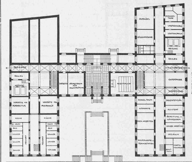
Sammlungsgebäude an der Sonneneggstrasse. — Erdgeschossgrundriss 1:800.
