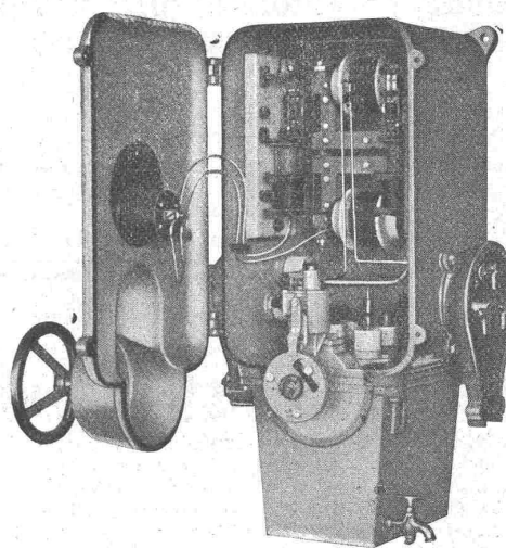
Type KH, 2000 Volt und 120 Ampère mit Min.-Max.-Auslösung, Freilauf und Ampèremeter.
