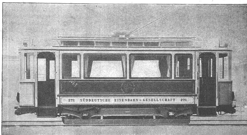
Motorwagen mit 20 Sitz- und 15 Stehplätzen. Typ: Mit Längssitzen, mittlere Seitenfenster herablassbar. Plattform mit vorderer Verglasung und seitlich mit Flügeltüren. vollständig abschliessbar; Radstand 3,2 m.
