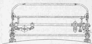
Abb. 27. Stromabnehmer. — 1:40.
