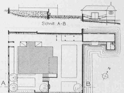
Abb. 1. Lageplan Villa Werdmüller. — 1 : 800.
