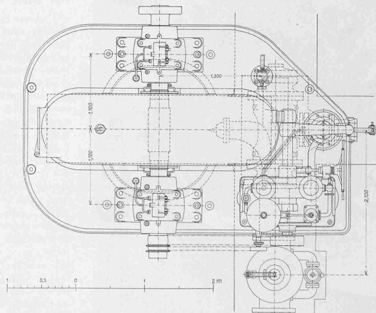
Abb. 19. Längsschnitt und Draufsicht der 6500 PS-Generatorturbine mit Schwenkdüse. Masstab 1 : 50. — Gebaut von Escher Wyss & Cie., Zürich.
