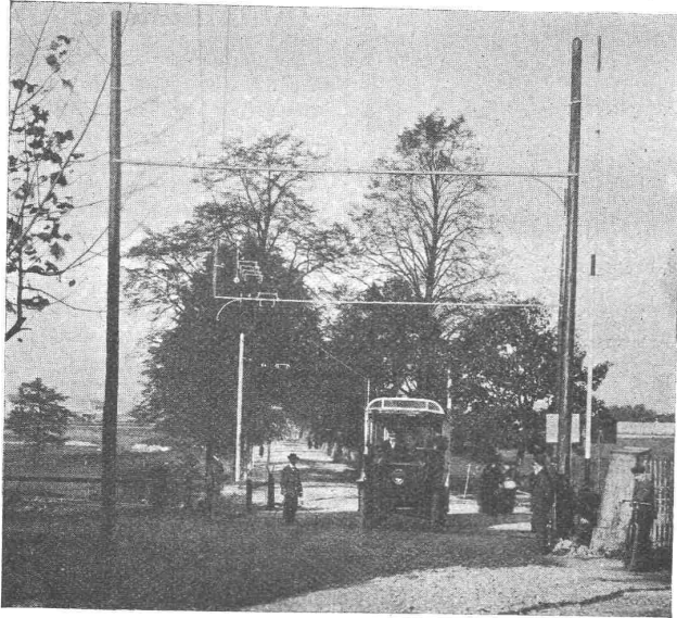
Linie Budweis in Böhmen. Niveau-Kreuzung mit der Hauptbahn Budweis-Prag.
